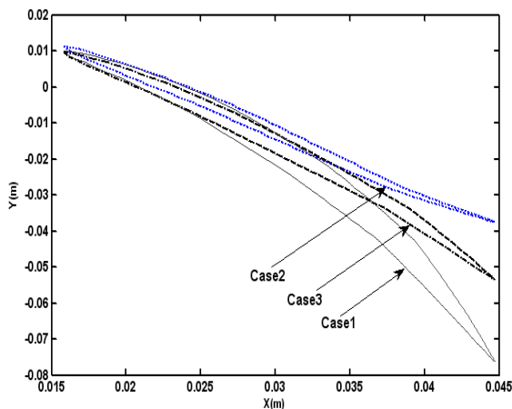
شکل (۲۰): مقطع ریشه پره روتور اول فن در بارگذاری‌های مختلف.
