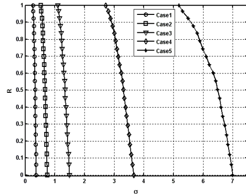
شکل (۲۹): توزیع ضریب صلبیت روتور طبقه اول فن در جهت شعاعی.
