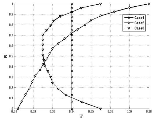
شکل (۱۶): توزیع ضریب بار روتور طبقه اول فن در جهت شعاعی.
