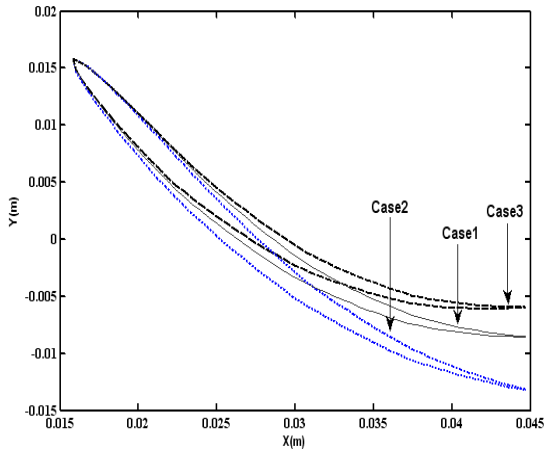
شکل (۱۹): مقطع نوک پره روتور طبقه اول در بارگذاری‌های مختلف.
