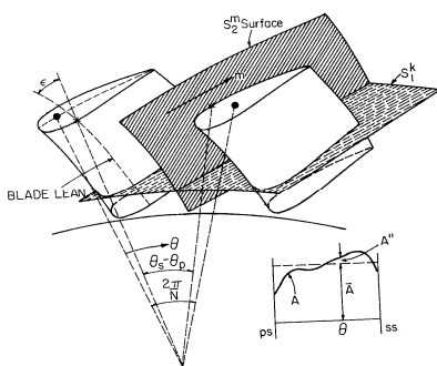
شکل (۱): صفحه‌های جريان S1 و S2.
