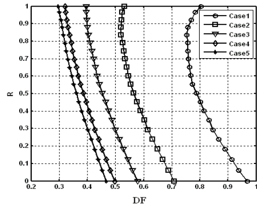
شکل (۲۸): توزیع ضریب پخش روتور طبقه اول فن در جهت شعاعی.
