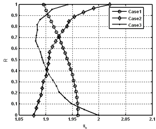
شکل (۱۷): توزیع نسبت فشار روتور طبقه اول فن در جهت شعاعی.
