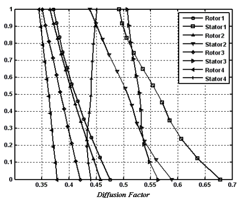
شکل (۱۵): توزیع ضریب پخش کمپرسور در جهت شعاعی.
