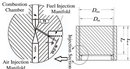
شکل (۱): شماتیک و جزئیات هندسه تزریق [۹].
