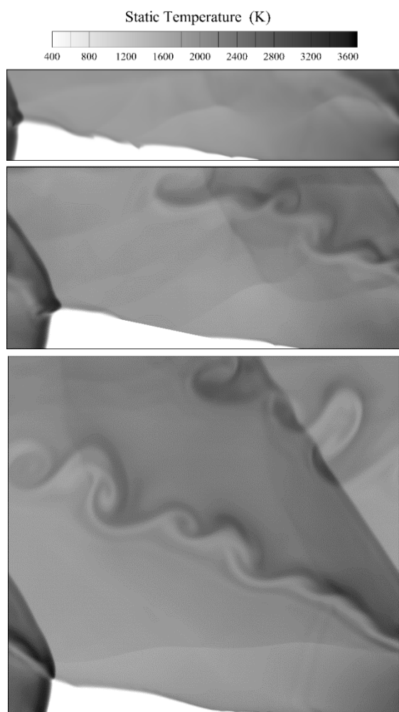
شکل (۱۰): کانتور دمای استاتیک برای طول مختلف محفظه.
