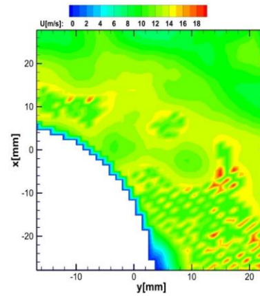
شکل (۱۷). میدان مؤلفه سرعت در جهت (x) سرعت بازسازی شده
