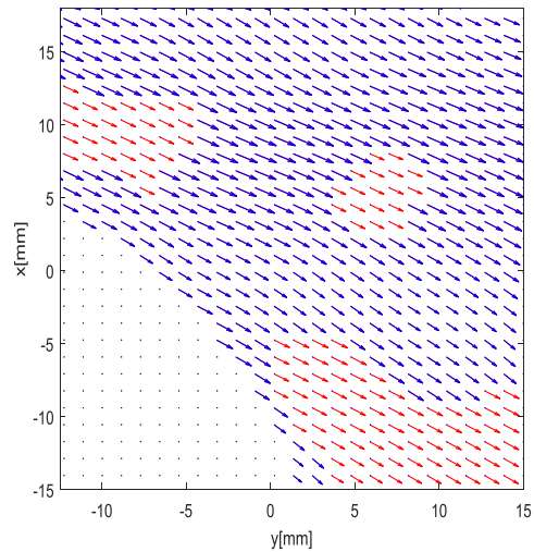
شکل (۹). نمایش تنهای بردارهای بازسازی در نقاط نقص میدان دویعدی سرعت
