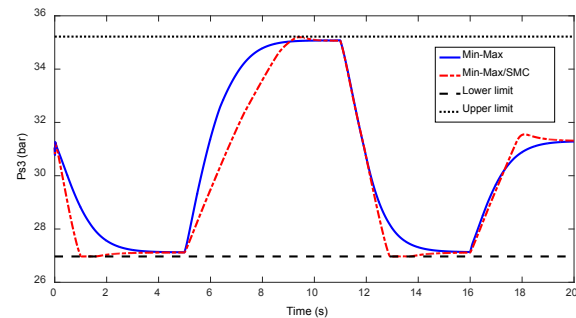
شکل (۱۳). پاسخ خروجی مقید Ps3
