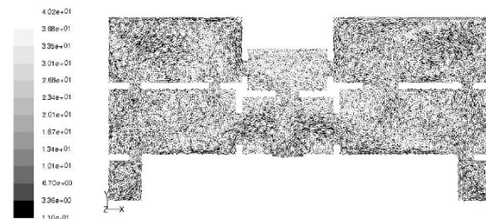
شکل (۲۰). بردار سرعت جریان هوا در ارتفاع ۱/۴m برحسب m/s بعد از مداخله ۲
