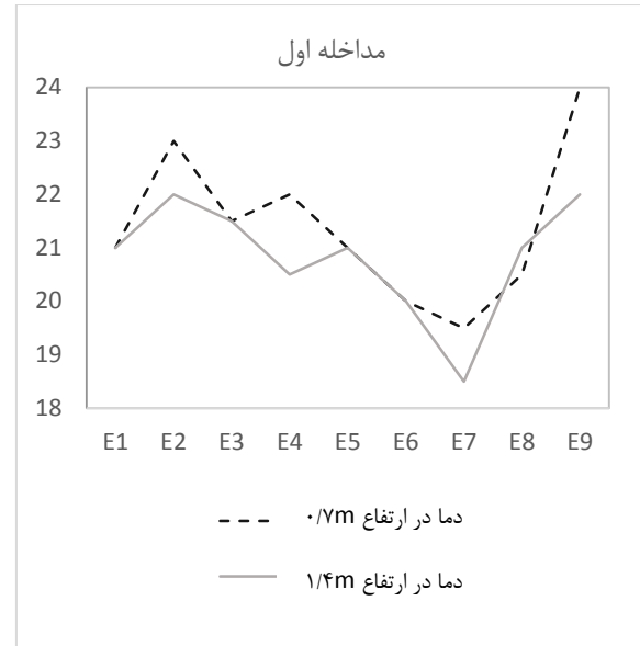
شکل (۱۸). دمای نقاط آزمون در محور E بعد از مداخله اول برحسب
