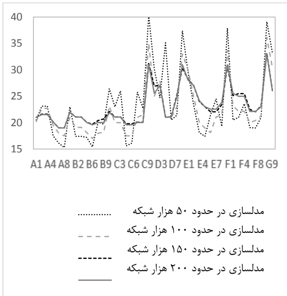
شکل (۷). مقایسه دمای شبیه‌سازی دما برحسب \square در ارتفاع 0/7\text{m} برای شبکه‌های مختلف
