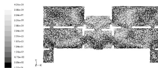
شکل (۱۵). بردار سرعت جریان هوا در ارتفاع ۱/۴m برحسب m/s بعد از مداخله ۱
