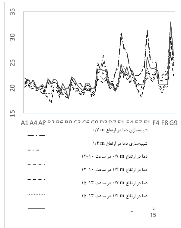
شکل (۶). مقایسه متوسط دمای آزمون تجربی و شبیه‌سازی برحسب \square
