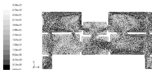
شکل (۱۱). بردار سرعت جریان هوا در ارتفاع ۰/۷m بر حسب طبق داده‌های تجربی
