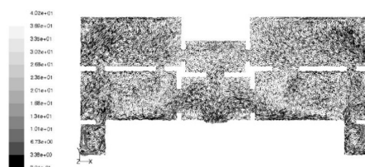
شکل (۲۷). بردار سرعت جریان هوا برحسب \text{m/s} بعد از مداخله ۳ در ارتفاع ۱/۴\text{m}
