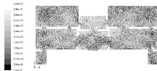
شکل (۱۹). بردار سرعت هوا در ارتفاع ۰/۷m برحسب m/s بعد از مداخله ۲
