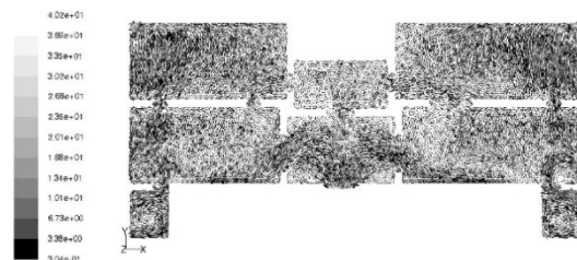
شکل (۲۶). بردار سرعت جریان هوا برحسب \text{m/s} بعد از مداخله ۳ در ارتفاع ۰/۷\text{m}
