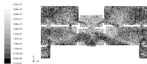
شکل (۱۴). بردار سرعت جریان هوا در ارتفاع ۷m برحسب m/s بعد از مداخله ۱
