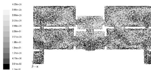
شکل (۳۲). بردارهای سرعت جریان هوا برحسب m/s از مداخله ۴ در ارتفاع ۱/۴m
