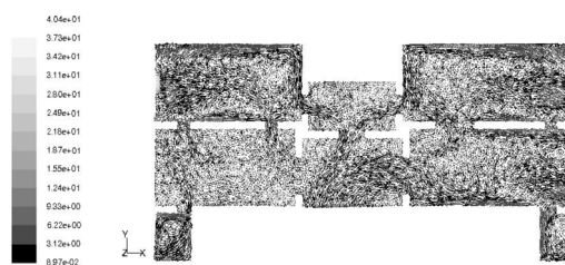
شکل (۱۰). بردار سرعت جریان هوا در ارتفاع ۱/۴m بر حسب طبق داده‌های تجربی
