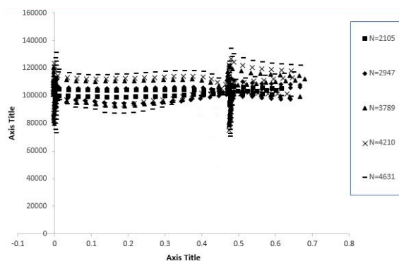
شکل (۷). نمودار تغییرات فشار طبقه کمپرسور تاندم دار بر حسب ۵۰٪ طول وتر پره در دورهای مختلف
