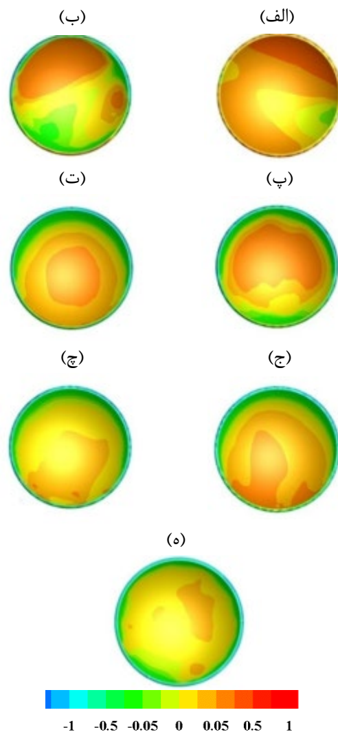
شکل (۷). توزیع فشار بر روی سطح جلویی سلول شماره ۱ برای سرعت ورودی ۱ متر بر ثانیه زاویه صفر تا 90^\circ درجه (از الف تا ه) با افزایش زاویه گام 15^\circ درجه
