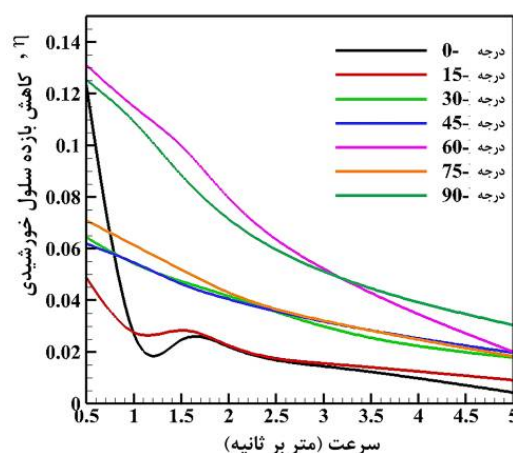
شکل (۱۵). مقایسه کاهش بازده روی سلول‌های سهموی برحسب سرعت در زوایای مختلف
