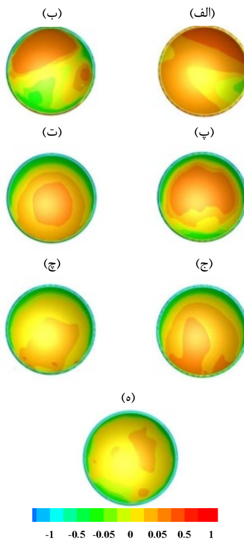
شکل (۷). توزیع فشار بر روی سطح جلویی سلول شماره ۱ برای سرعت ورودی ۱ متر بر ثانیه زاویه صفر تا 90 درجه (از الف تا ه) با افزایش زاویه گام 15 درجه
