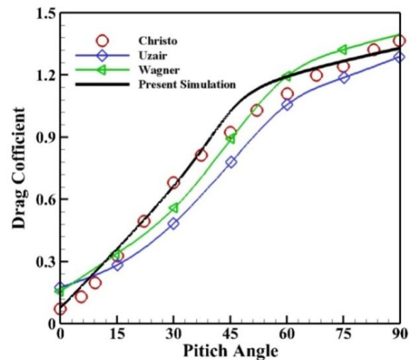
شکل (۴). مقایسه تغییرات ضریب پسا برحسب زاویه گام حاصل از پژوهش حاضر با داده‌های گزارش شده برای سرعت جریان ۳/۲ متر بر ثانیه [۹ و ۸]
