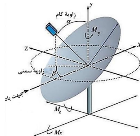
شکل (۹). ساختار کلی یک سلول سهموی به سبک دایره کامل
