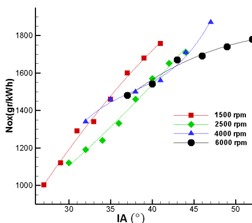
شکل (۵): تولید آلاینده اکسیدهای نیتروژن به ازاء مقادیر مختلف آوانس جرقه در شرایط تمام بار و حالت گازسوز
