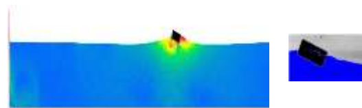
(ب) 7/2 s، راست تصویر آزمایشگاهی و چپ‌نمای شبیه‌سازی
