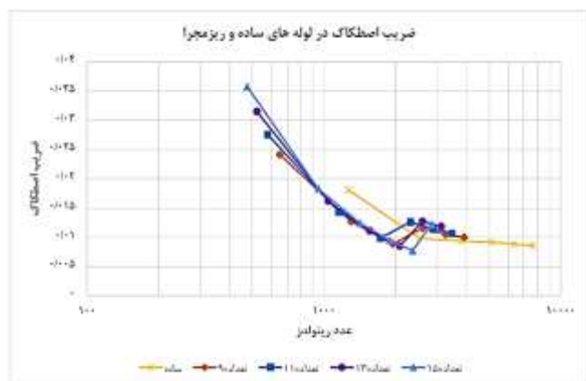
شکل (۱۳): ضریب اصطکاک در لوله‌های ساده و ریزمجرا
