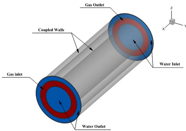
شکل (۴): شرایط مرزی مبدل حرارتی سه لوله‌ای
