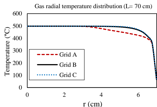
شکل (۲): توزیع شعاعی دمای دود در خروجی مبدل حرارتی
