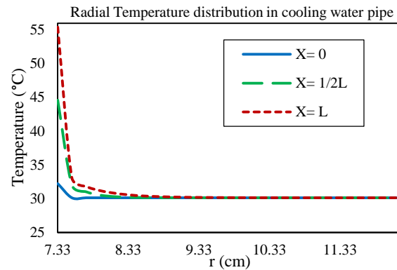
شکل (۳): توزیع شعاعی دمای آب سرد در پوسته بیرونی در سه مقطع از مبدل حرارتی دو لوله‌ای
