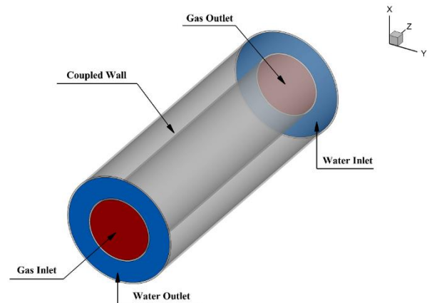
شکل (۱): شرایط مرزی مبدل حرارتی دو لوله ای
