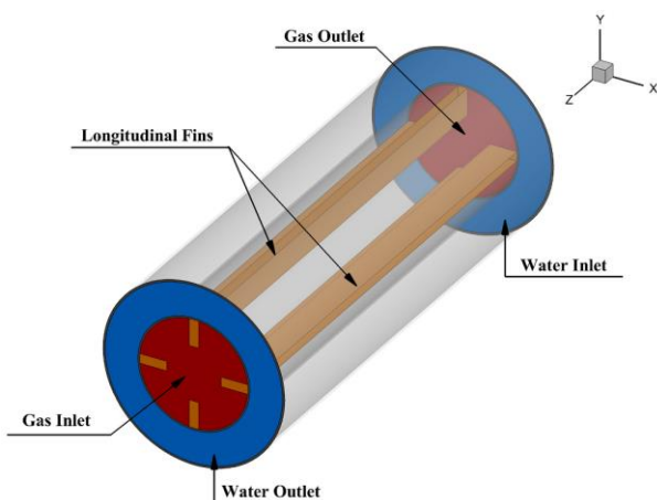
شکل (۷): شرایط مرزی مبدل حرارتی با پره‌های طولی
