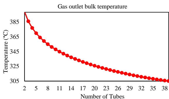
شکل (۸): دمای متوسط گاز خروجی بر حسب تعداد لوله‌های مبدل حرارتی پوسته و لوله
