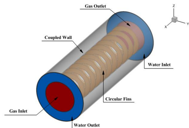
شکل (۶): شرایط مرزی مبدل حرارتی با پره‌های حلقوی (Case D)
