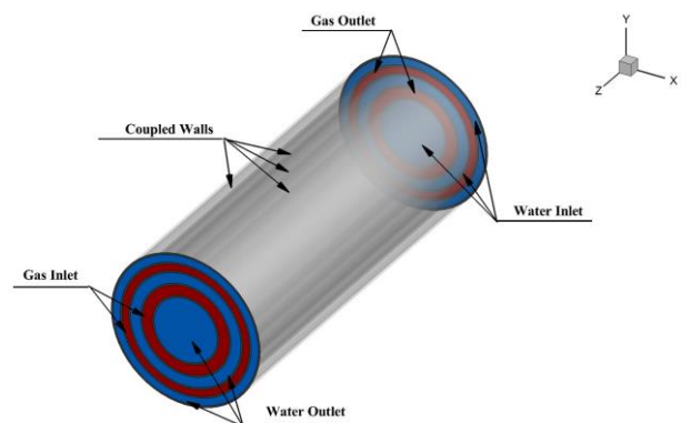
شکل (۵): هندسه مبدل پنج لوله‌ای
