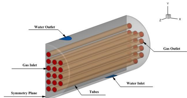
شکل (۹): شرایط مرزی مبدل پوسته و لوله ۳۰ لوله‌ای
