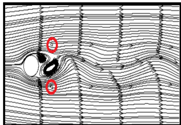
ب) کنترل کننده در X=0.137 m
