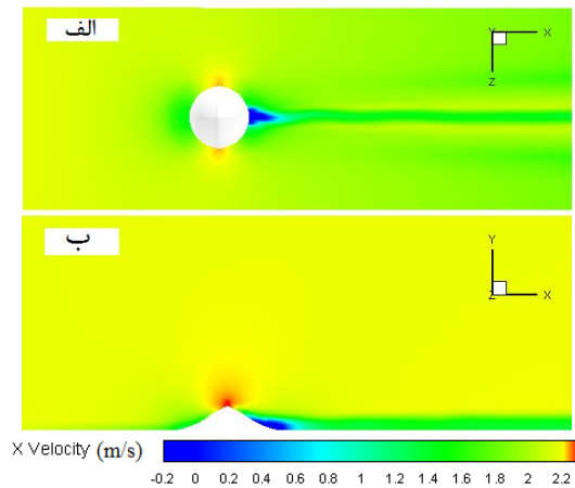
شکل (۴): خطوط هم‌تراز مؤلفه افقی سرعت در زمان ۱۰ روی (الف) صفحه Y = 0.05 m (ب) Z = 0 m
