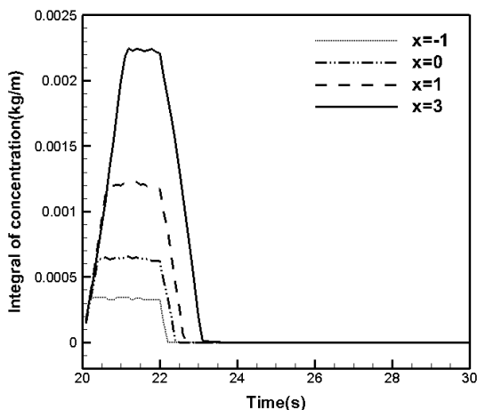
شکل (۸): تغییرات انتگرال سطحی غلظت روی سطح زمین بر حسب زمان روی صفحات عمود بر جهت جریان
