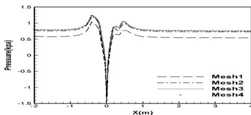
شکل (۲): بررسی استقلال حل از شبکه بر اساس توزیع
