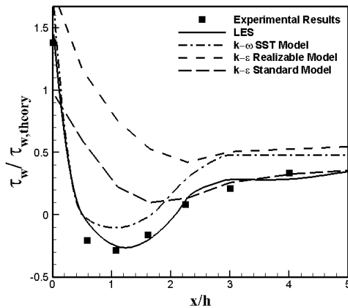
شکل (۳): مقایسه تغییرات تنش برشی بی‌بعد شده روی سطح تپه با نتایج آزمایشگاهی حاصل از رویکردهای مختلف مدل‌سازی آشفتگی [۱۲]
