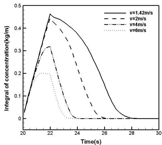
شکل (۷): تغییرات انتگرال سطحی غلظت روی سطح زمین بر حسب زمان به ازای سرعت‌های مختلف جریان ورودی
