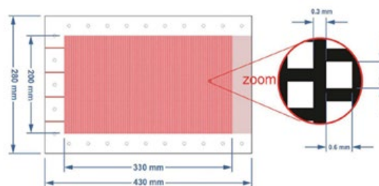
شکل ۴. طراحی محیط متخلخل مورد استفاده در پژوهش حاضر
