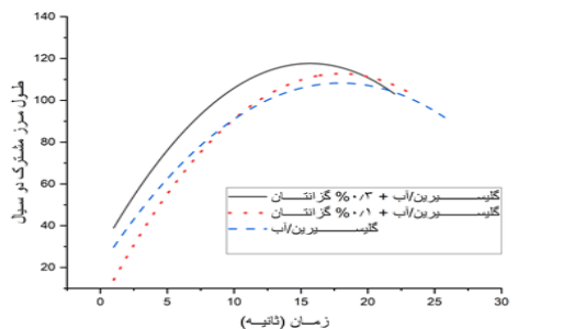
شکل ۶. تغییرات پارامتر طول مرز مشترک با گذشت زمان در طول سلول برای سیال مختلف پر شده محیط متخلخل
