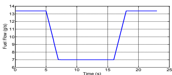
شکل (۱۵): برنامه سوخت موتور برای تحلیل عملکرد گذرا
