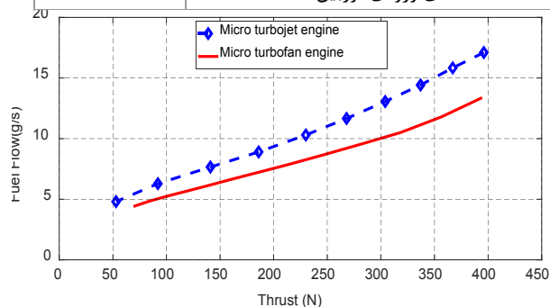
شکل (۱۸): مقایسه عملکرد موتور میکرو-توربوفن و میکرو-توربوجت پایه
