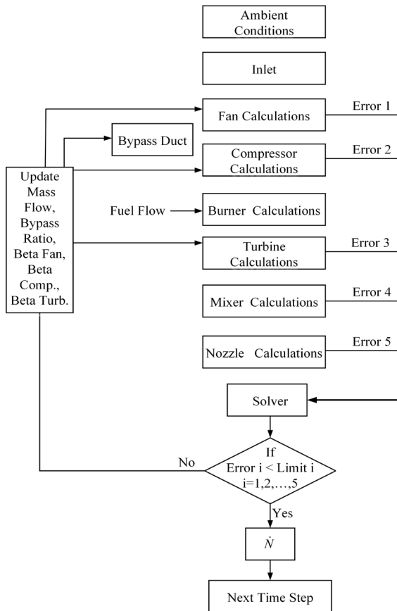
شکل (۵): روش تکرار ماتریسی برای مدل سازی
