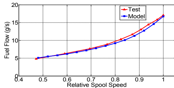
شکل (۳): سوخت موتور پایه برحسب دور نسبی شفت
