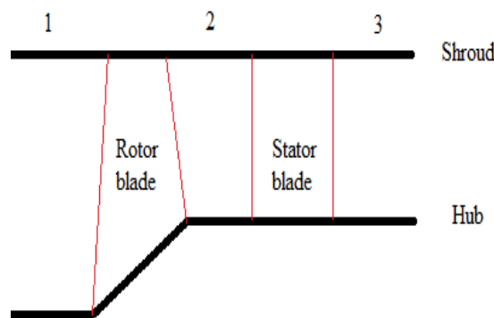
شکل (۸): شماتیک فن طراحی شده
