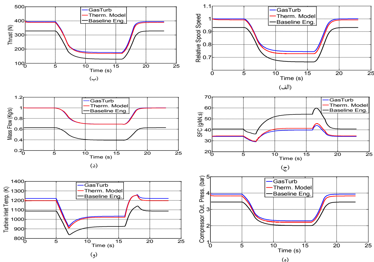
شکل (۱۶): عملکرد موتور میکرو-توربوفن در سناریوی گذرا: (الف) سرعت نسبی شفت، (ب) تراست، (ج) مصرف سوخت ویژه، (د) دبی هوای ورودی، (ه) فشار خروجی کمپرسور، (و) دمای ورودی توربین
