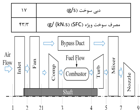
شکل (۱): شماتیک اجزای موتور میکرو-توربوفن با جریان آمیخته
