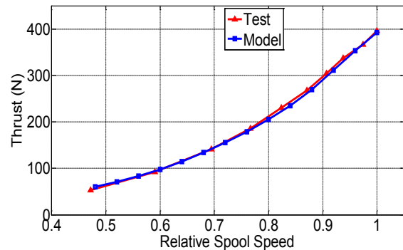
شکل (۲): تراست موتور پایه برحسب دور نسبی شفت
