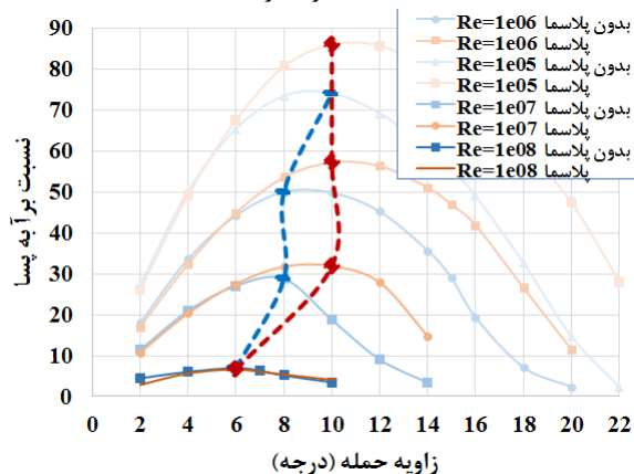
شکل (۱۴): نسبت برآ به پسا بر حسب زاویه حمله به ازای اعداد رینولدز مختلف (تغییرات لزجت)
