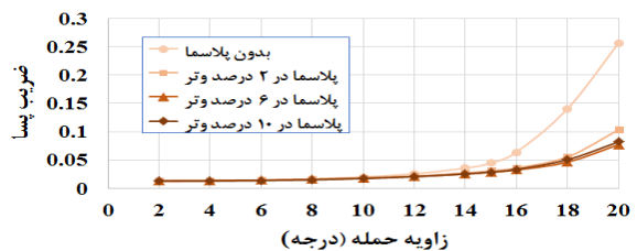
شکل (۹): ضریب پسا بر حسب زاویه حمله به ازای جانمایی مختلف پلاسما
