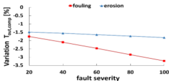
شکل (۱۵): تاثیر رسوب‌گذاری و فرسایش پره‌های کمپرسور بر دمای خروجی کمپرسور
