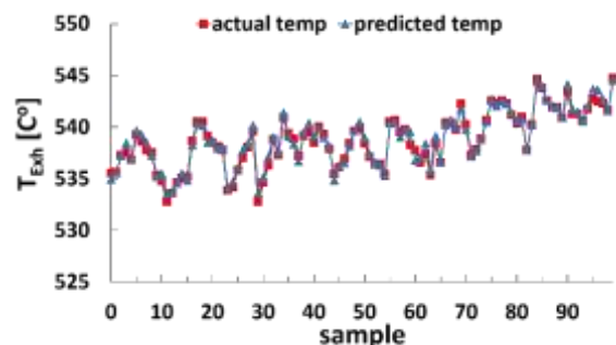
شکل (۸): مقایسه دمای واقعی و پیش‌بینی شده خروجی از توربین
