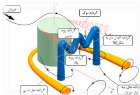
شکل (۱): فیزیک جریان حول استوانه محدود [۱۰]
