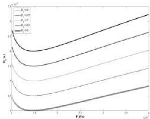
شکل (۷): تغییرات قطر خروجی نازل بر اساس تغییرات فشار ورودی پیشران و تغییرات قطر گلوبی نازل
