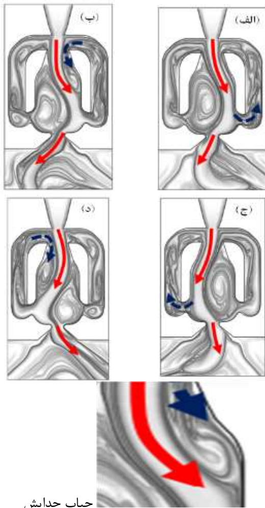
شکل (۱): طریقه عملکرد نوسان‌سازهای سیال متصل به دیوار [۷]
