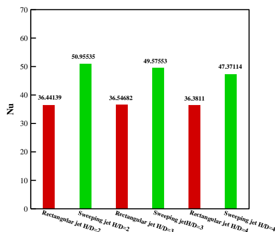
شکل (۱۱): نمودار عدد ناسلت میانگین در فواصل مختلف برای جت نوسانی و جت ثابت در Re=8000 و \tau = \frac{T_f}{\rho}
