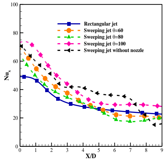
شکل (۱۴): نمودار عدد ناسلت در زوایای نازل مختلف برای جت نوسانی و جت ثابت در Re=8000 و H=3D
