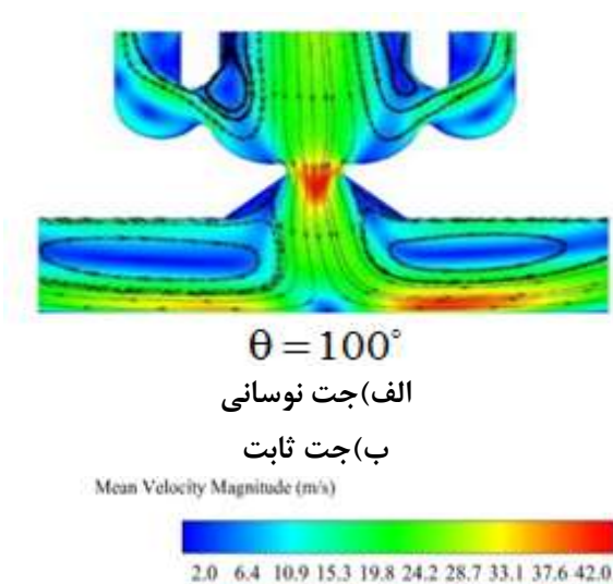
شکل (۱۷): توزیع سرعت در زوایای نازل مختلف برای جت
