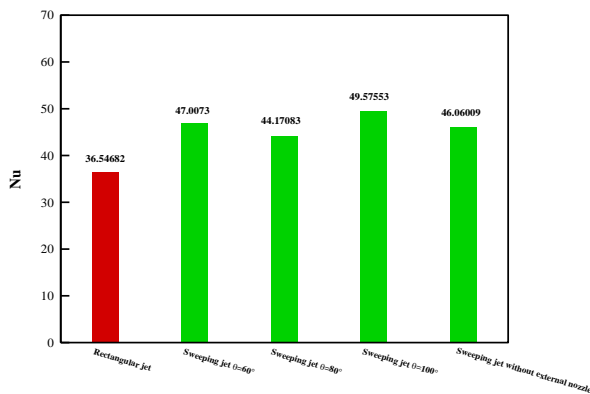
شکل (۱۵): نمودار عدد ناسلت میانگین در زوایای نازل مختلف برای جت نوسانی و جت ثابت در Re=8000 و H=3D
