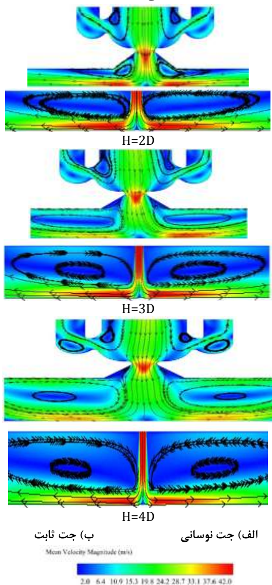
شکل (۱۲): نمودار سرعت مقطع X=3D در فواصل H=2D و H=3D برای جت نوسانی در Re=8000 و \tau = \frac{T_f}{\rho}
