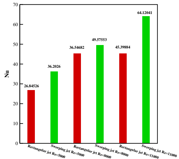
شکل (۱۹): نمودار عدد ناسلت میانگین در اعداد رینولدز
