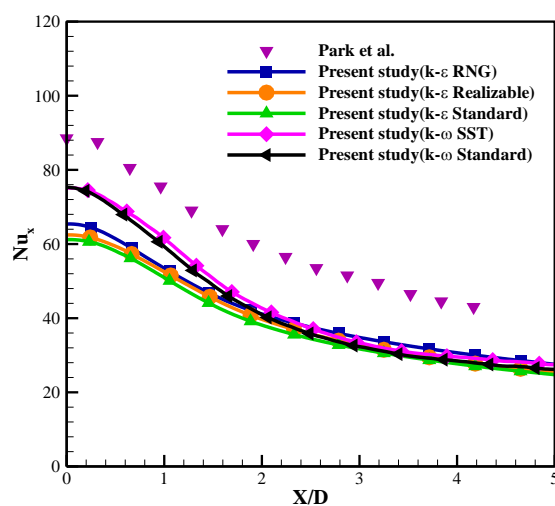
شکل (۸): بررسی مدل‌های جریان آشفته مختلف برای جت نوسانی
