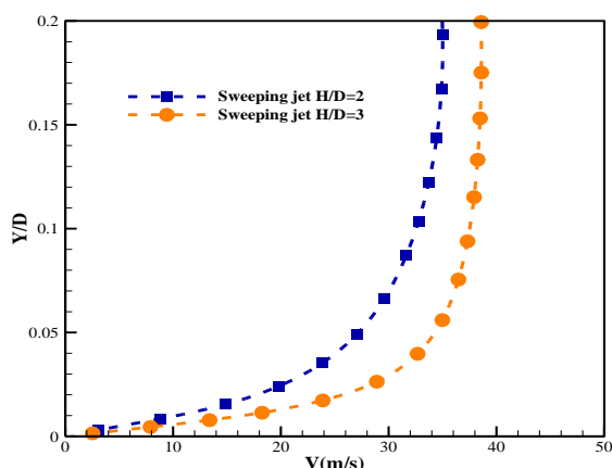
شکل (۱۲): نمودار سرعت مقطع X=3D در فواصل H=2D و H=3D برای جت نوسانی در Re=8000 و \tau = \frac{T_f}{\rho}
