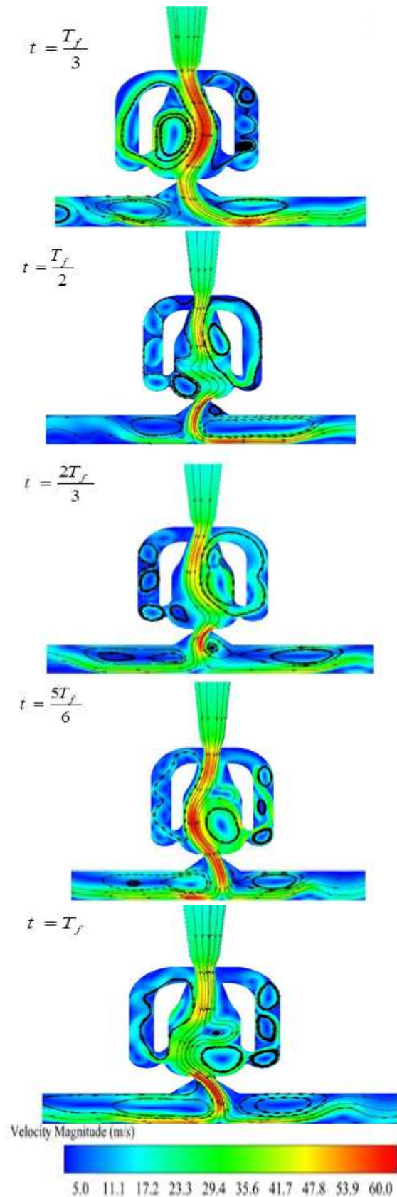
شکل (۹): کانتور سرعت در یک دوره تناوب برای جت نوسانی Re=8000 و \theta = 100^\circ و H/D=3 در
