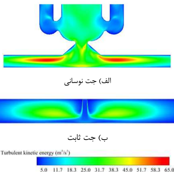
شکل (۲۱): توزیع انرژی جنبشی آشفتگی برای جت نوسانی و جت ثابت در Re=8000 , H=2D و \theta = 100^\circ
