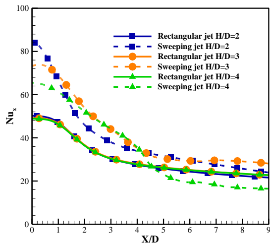
شکل (۱۰): نمودار عدد ناسلت در فواصل مختلف برای جت نوسانی و جت ثابت در Re=8000 و \tau = \frac{T_f}{\sigma}
