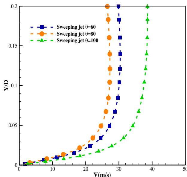
شکل (۱۶): نمودار سرعت مقطع X=3D در زوایای نازل
