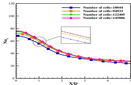
شکل(۸): نمودار استقلال از شبکه جت نوسانی
