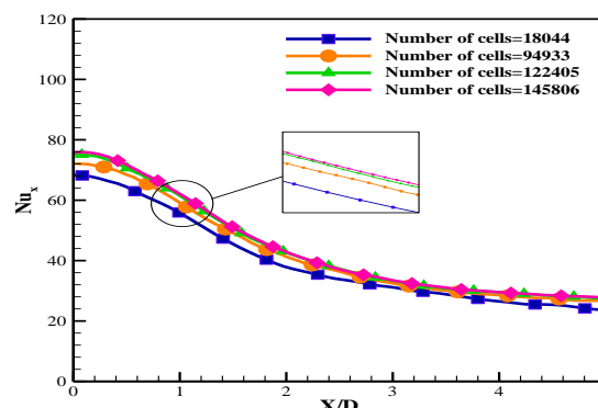
شکل (۵): نمودار استقلال از شبکه جت نوسانی
