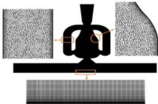
شکل (۴): نمایی از شبکه بندی نوسان ساز سیال
