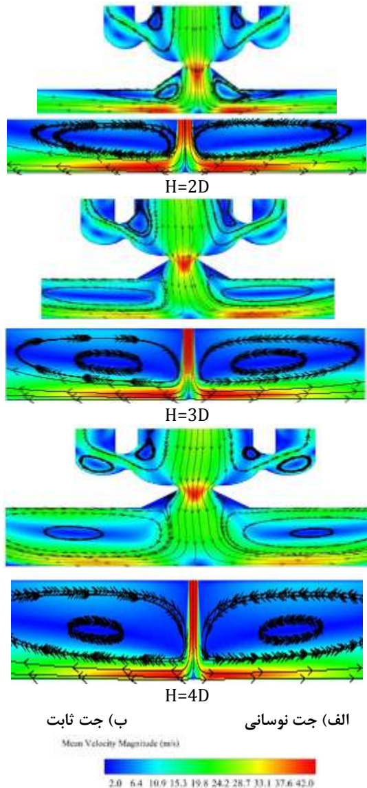
شکل (۱۳): توزیع سرعت در فواصل مختلف برای جت نوسانی و جت ثابت در Re=8000 و \tau = \frac{T_f}{\sigma}
