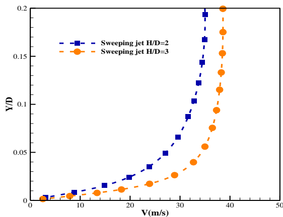
شکل (۱۲): نمودار سرعت مقطع X=3D در فواصل H=2D و H=3D برای جت نوسانی در Re=8000 و \tau = \frac{T_f}{\sigma}
