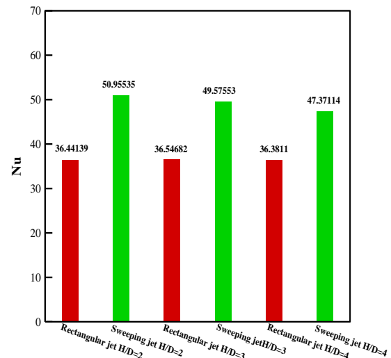
شکل (۱۱): نمودار عدد ناسلت میانگین در فواصل مختلف برای جت نوسانی و جت ثابت در Re=8000 و \tau = \frac{T_f}{\sigma}
