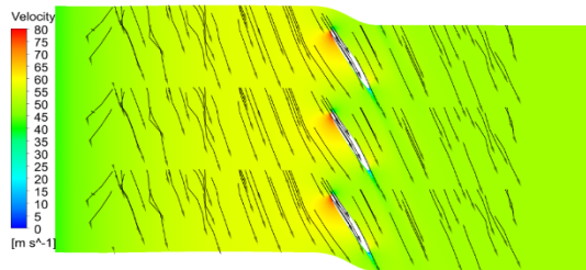
شکل (۱۳): بردارهای سرعت در نمای تیغه به تیغه و در ۵۰٪ طول تیغه
