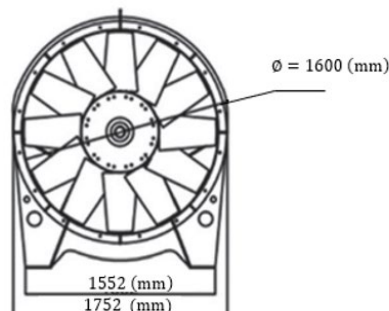
شکل (۱): هندسه فن مورد مطالعه [۸]
