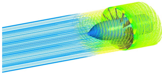
شکل (۱۱): خطوط جریان در دبی حجمی ثابت Q=30 \text{ (m}^3/\text{s)}
