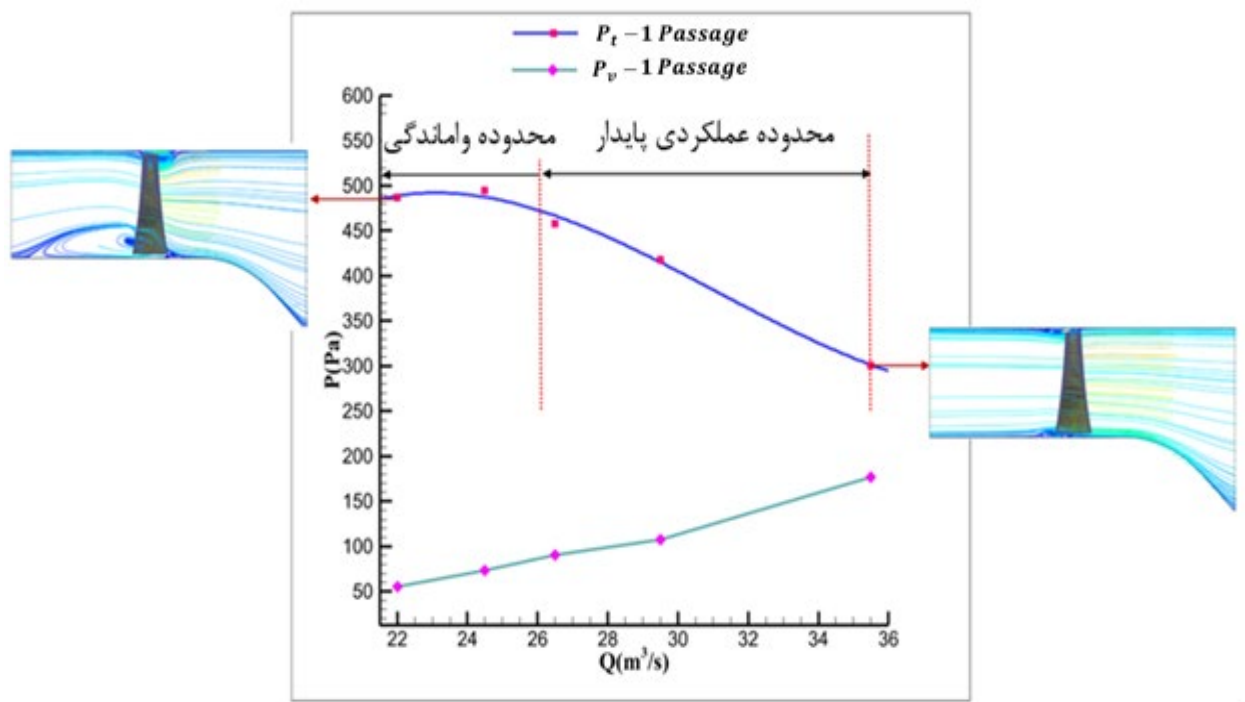
شکل (۱۷): محدوده‌های عملکردی پایدار و ناپایدار فن و خطوط جریان متناظر
