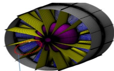
مش تولید شده روی تیغه و سطح تویی
