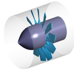
شکل (۳): نمای ایزومتریک فن به همراه مش تولید شده در یک گذرگاه
